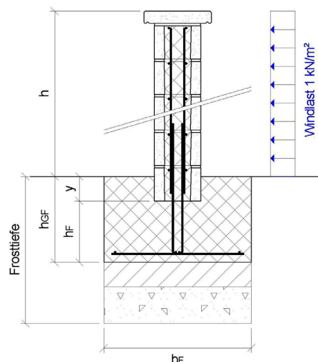
Bild 21: Schematische Darstellung einer freistehenden Mauer, Annahme Windlast 1 kN/m 2 , mit Bewehrungseinlagen (technische Werte siehe Tabelle 12)
