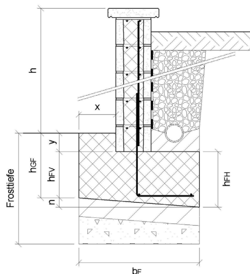
Bild 23: Schematische Darstellung einer Mauer mit horizontaler Hinterfüllung ohne zusätzliche Auflast, mit Bewehrungseinlagen (technische Werte siehe Tabelle 14)
