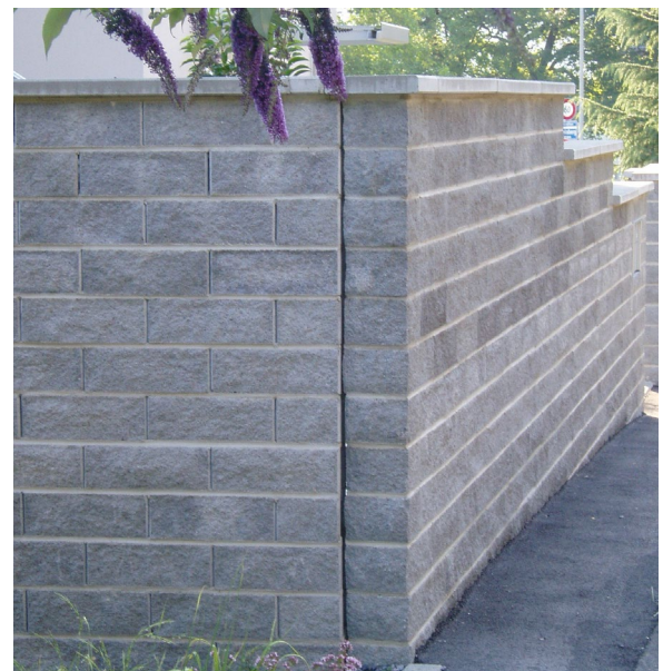
Bild 41: Dilatationsfuge (Produktneutral)
