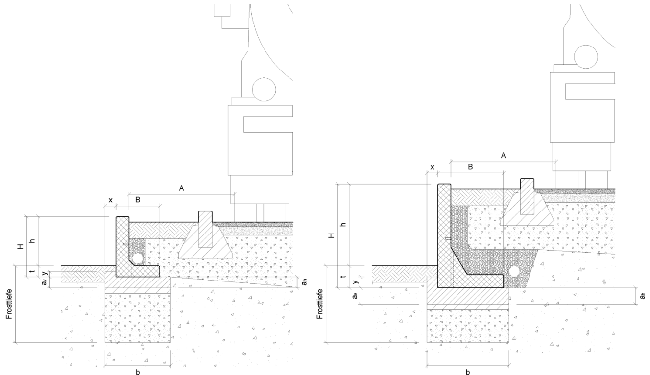
Bild 35: Fundamentabmessungen für Lastfall C4, A = 70 cm
