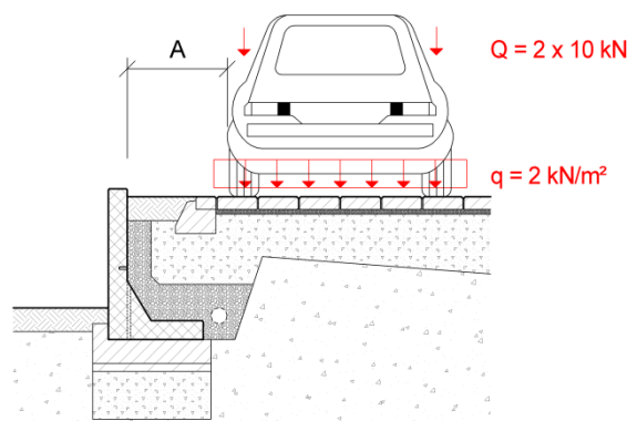
Bild 9: Lastfall B2
