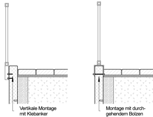
Bild 32: Mögliche Montagen von Geländer
