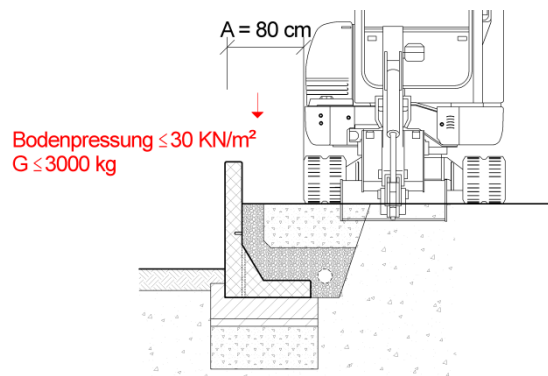
Bild 14: Lastfall G2
