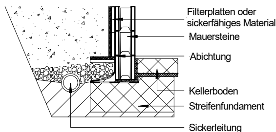
Bild 18 Entwässerung
