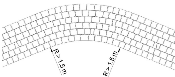
Réalisation de courbes avec les pavés FRIEDA®.
