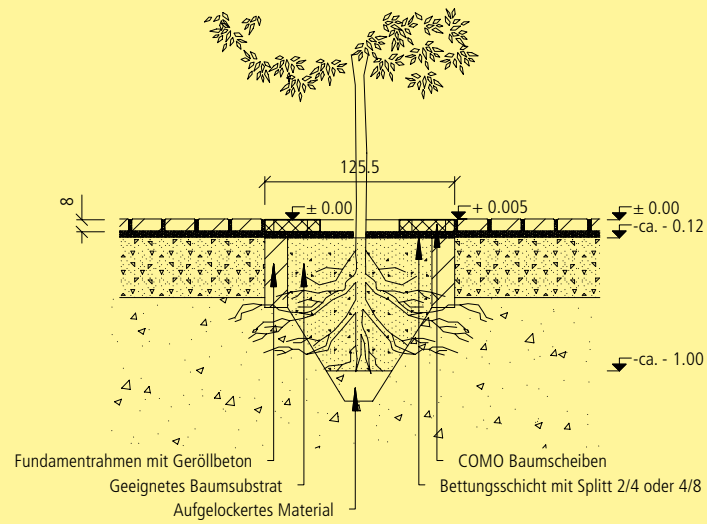
Einbauschema COMO Baumscheiben mit Fundamentrahmen (bauseits)
