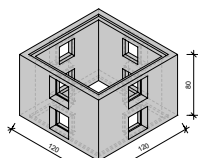
Type 1, B 120cm L 120cm H 80cm
