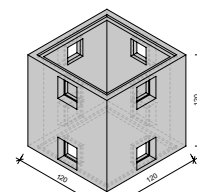
Type 1, B 120cm L 120cm H 120cm
