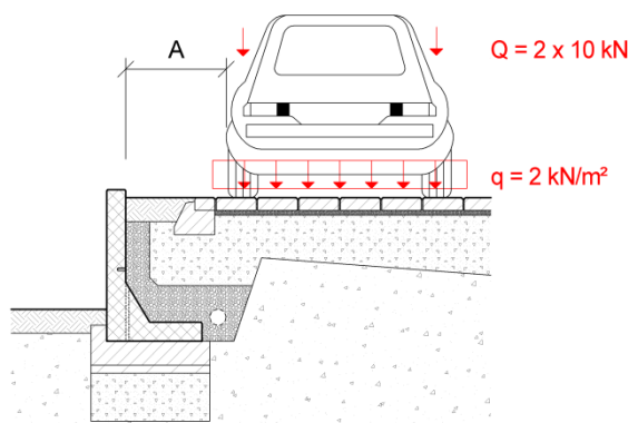
Bild 9: Lastfall B2
