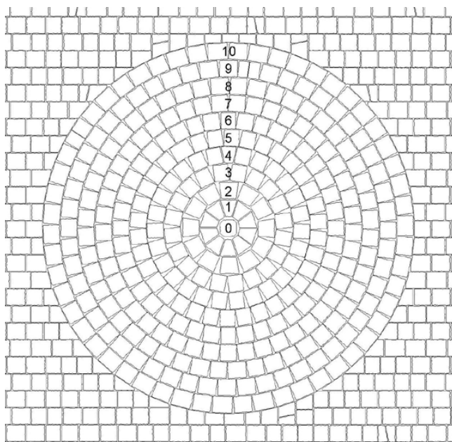
Pavage circulaire avec les pavés FRIEDA®
