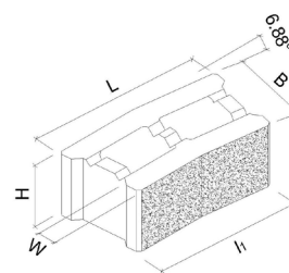
Bild 11: Radiusspaltsteine, 2-seitig gespalten
