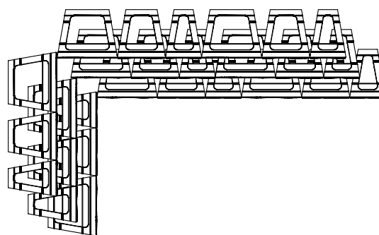
Illustration 15 : plan d'angle intérieur avec un retrait de 16,5 cm
