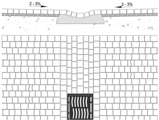
Possibilité de réalisation de cunette avec des pavés FRIEDA®
