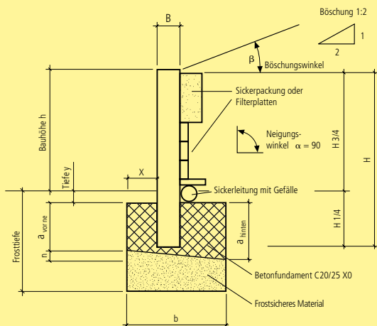
Palisadeneinbau
