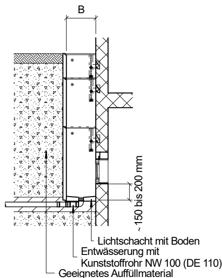
Bild 29: Lichtschachtssole mit Boden: z.B. Entwässerung an Meteorleitung
