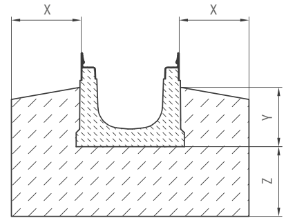
Présentation avec caniveau type BIRCOslim®
