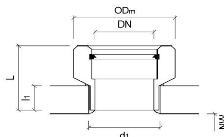
Bild 2: CENTUB® Klebeanschlussstück 90°
