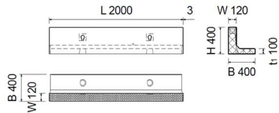
Illustration 8 : Bordures de quai de type 8
