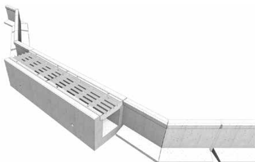
Photo 1 : représentation schématique du caniveau-barrière amphibien
