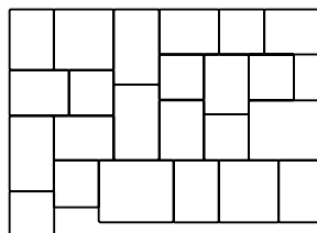
Verlegemuster 2 Wilder Verband, Randabschluss zuschneiden
