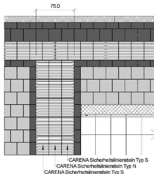
Bild 15: Anordnung von Aufmerksamkeitsfeldern mit einer Breite von 75 cm mit Steinen H = 8 cm
