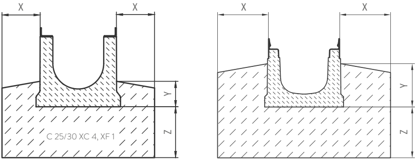
Montage suivant catalogue des structures types de chaussées avec de couches de fondation anti-gel (composition libre)
