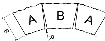
Bild 34: Muffenöffnungen bei Radien R > 58 cm bei Steinen mit B = 20 cm bzw. R > 56 cm bei Steinen mit B = 25 cm
