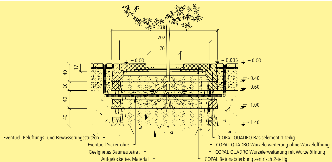
Einbauschema COPAL QUADRO Baumwurzelschutz mit Betonabdeckung exzentrisch und Wurzelerweiterung mit Wurzelöffnungen
