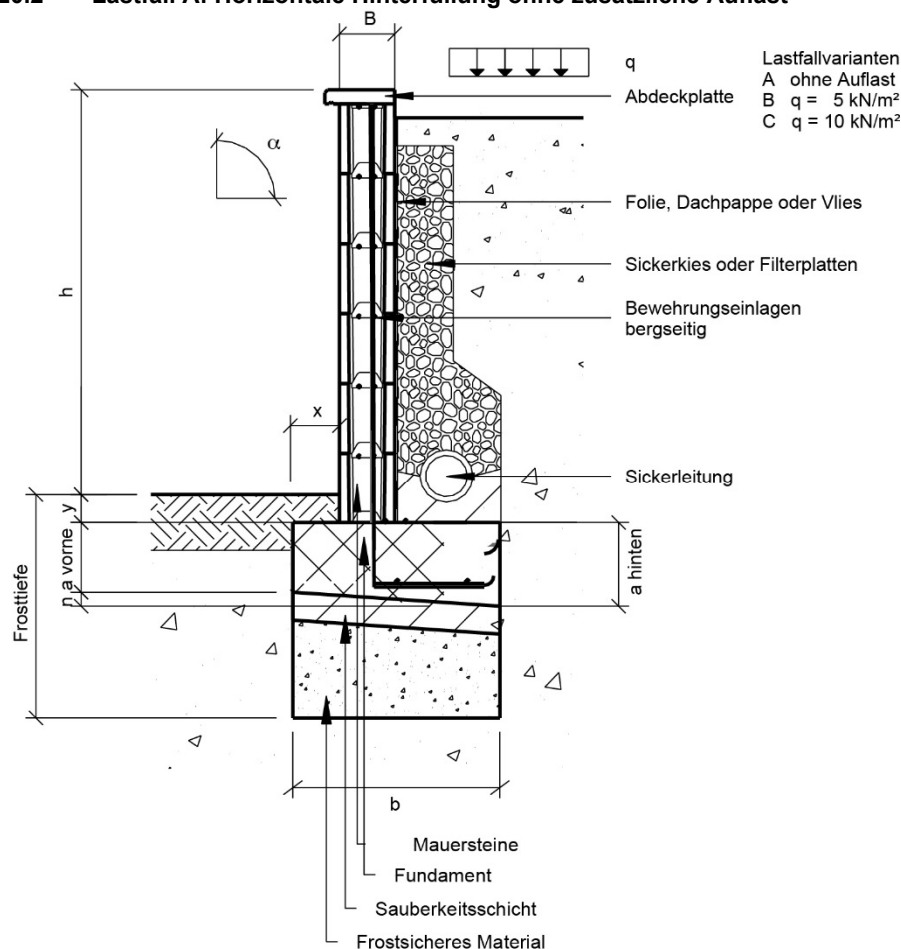
Bild 20: Maueraufbau horizontale Hinterfüllung ohne zusätzliche Auflast
