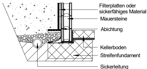
Bild 18 Entwässerung
