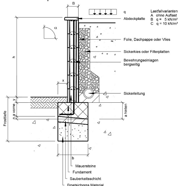
Bild 9: Aufbauquerschnitt mit Bewehrungsmöglichkeit
