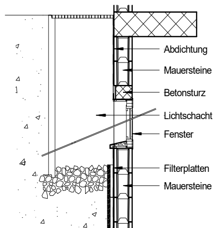
Bild 17: Querschnitt: Kellerwand mit Fenster und Betonsturz
