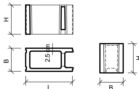
Bild 6: SCHALIT Endstein
