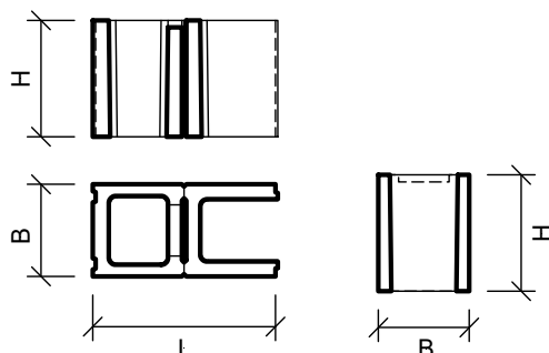
Bild 8: SCHALIT Trenn- und Endstein
