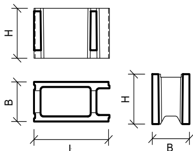
Bild 4: SCHALIT Normalstein
