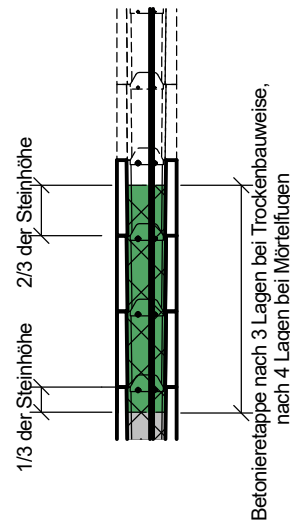
Bild 10: Betonieretappen
