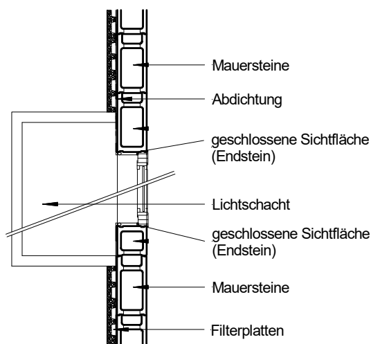
Bild 16: Grundriss: Kellerwand mit Fenster
