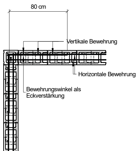
Bild 14: Eckausbildung
