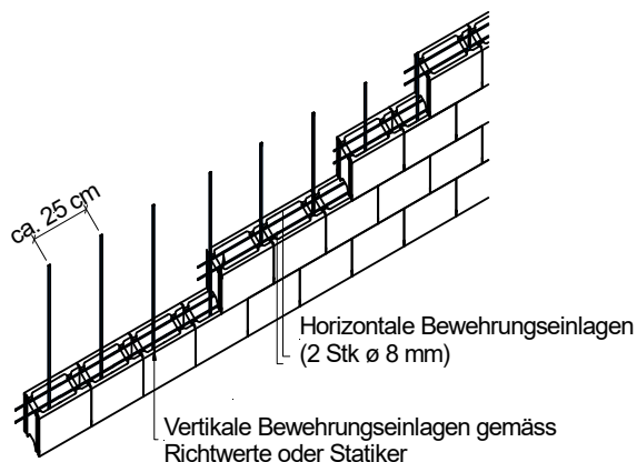
Bild 13 Maueraufbau mit Bewehrung
