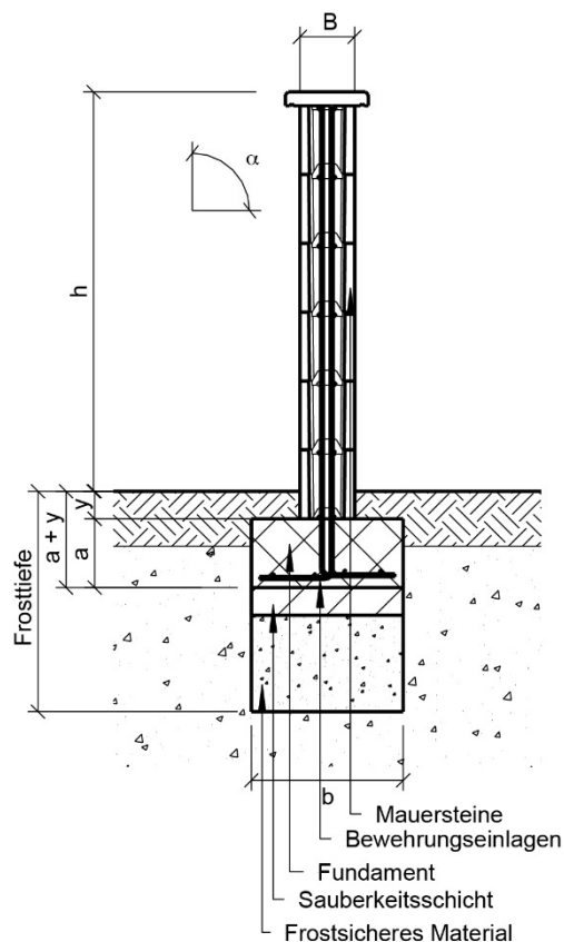
Bild 19: Maueraufbau freistehend, Windlast 1 kN/m 2
