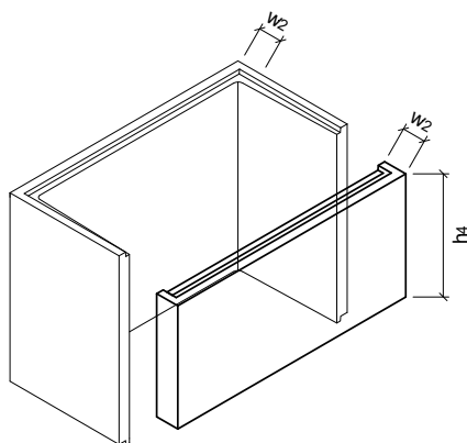
Bild 10: Zusatzwand
