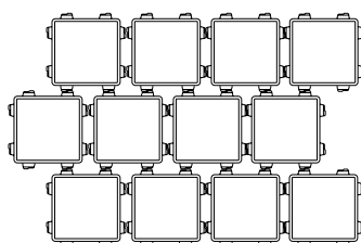
Englischverbund
