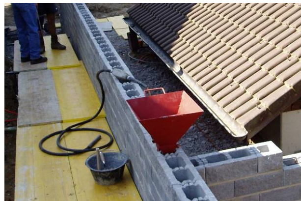
Bild 50: Einbringen von Füllbeton mit einem geeigneten Trichter
