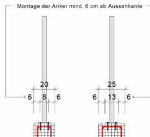
Montages possibles de garde-corps
