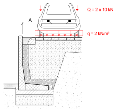
Bild 12: Lastfall B2
