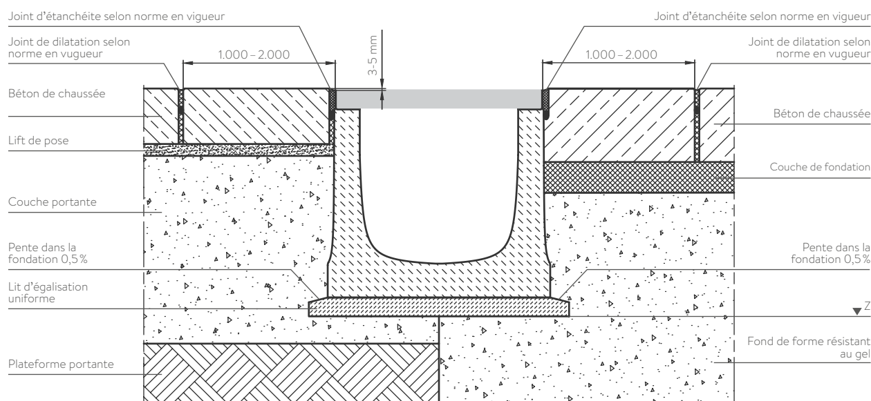
Montage suivant catalogue des structures types de chaussées avec de couchés de fondation anti-gel (composition libre)
