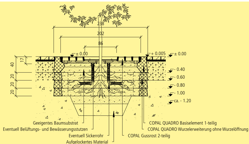
Einbauschema COPAL QUADRO Baumwurzelraumschutz mit Gussrost und Wurzelerweiterung ohne Wurzelöffnungen
