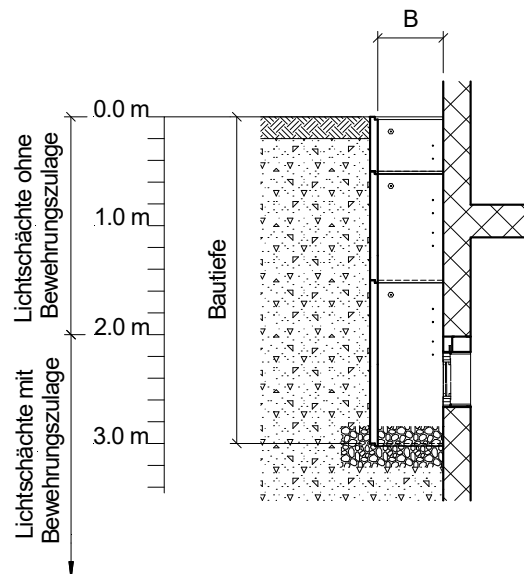
Bild 18: Lastfall A, horizontale Hinterfüllung ohne zusätzliche Auflast
