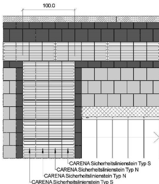
Bild 16: Anordnung von Aufmerksamkeitsfeldern mit einer Breite von 100 cm mit Steinen H = 8 cm
