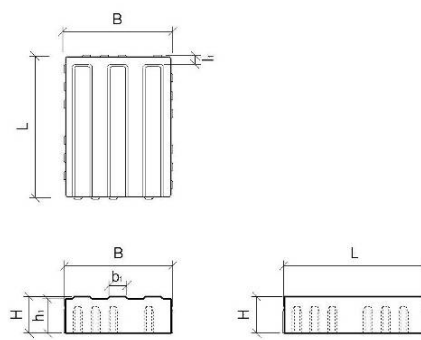
Bild 4: CARENA® Sicherheitslinienstein Typ S; H 6 cm
