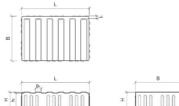
Bild 6: CARENA® Sicherheitslinienstein Typ S; H 8 cm
