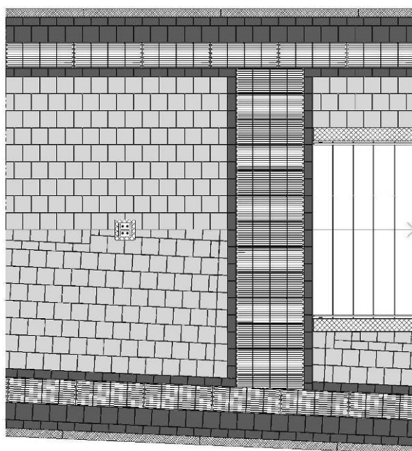
Bild 21: Anordnung mit CARENA® Pflastersteinen bei geraden nicht parallel verlaufenden Perronkanten
