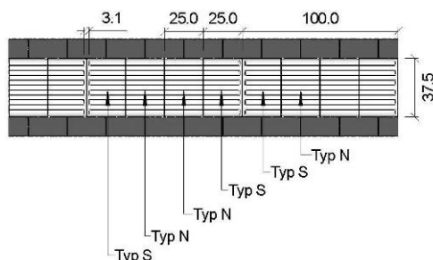
Bild 12: Gestaltung der Sicherheitslinien mit Steinen H = 8 cm
