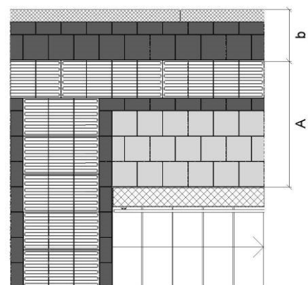
Bild 10: Definition Abstand A
