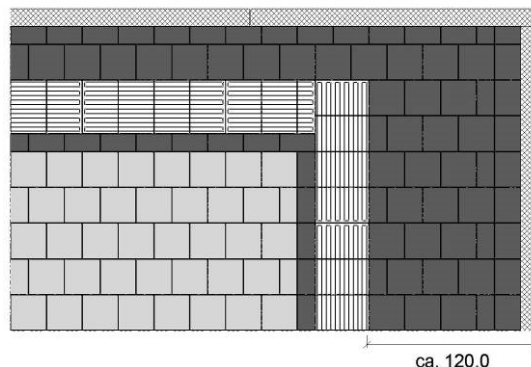
Bild 14: Anordnung beim Ende einer Perronanlage
