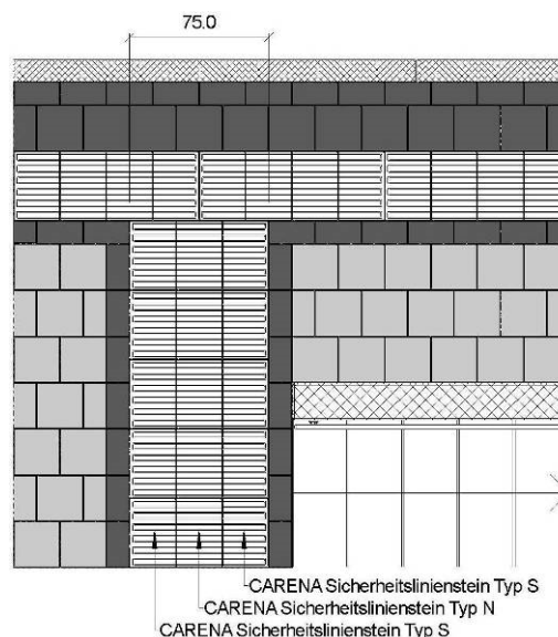
Bild 15: Anordnung von Aufmerksamkeitsfeldern mit einer Breite von 75 cm mit Steinen H = 8 cm
