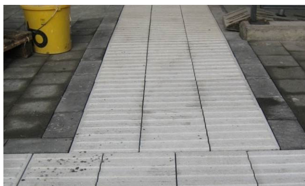
Bild 18: Anschluss Aufmerksamkeitsfelder an Sicherheitslinie
