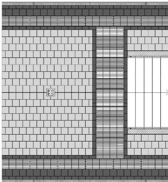
Bild 20: Anordnung mit CARENA® Pflastersteinen bei geraden parallel verlaufenden Perronkanten
