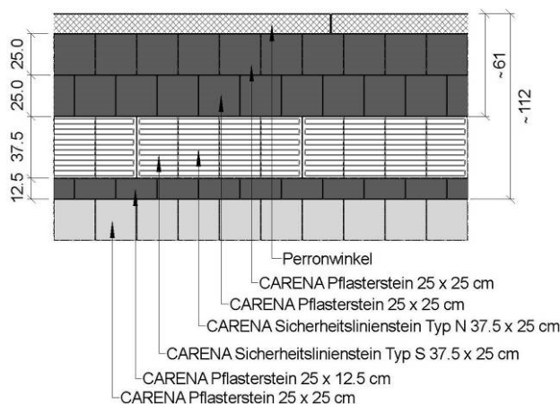
Bild 8: Anordnung als Beispiel bei Durchfahrtsgeschwindigkeiten V_R 101 bis 120 km/h oder V_A 91 bis 100 km/h ( b \sim 61 cm) bei der Verwendung von CARENA® Pflastersteinen H = 8 cm
