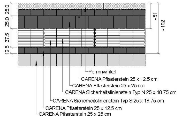
Bild 9: Anordnung als Beispiel bei Durchfahrtsgeschwindigkeiten V_R bis 100 km/h oder V_A bis 90 km/h ( b \sim 51 cm) bei der Verwendung von CARENA® Pflastersteinen H = 6 cm
