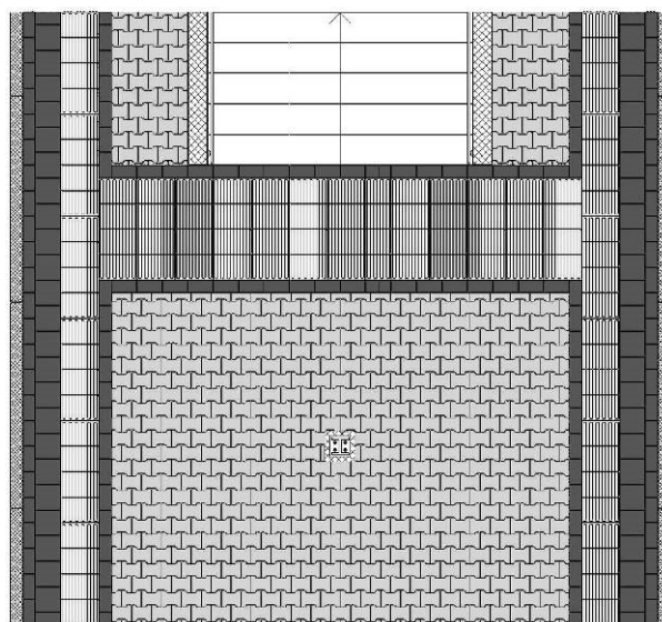
Bild 22: Anordnung mit CARENA® Pflastersteinen bei bestehenden Pflastersteinen
