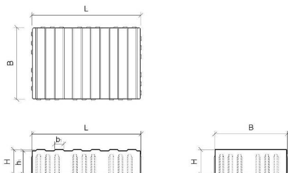
Bild 5: CARENA® Sicherheitslinienstein Typ N; H 8 cm
