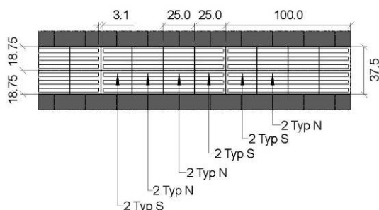
Bild 13: Gestaltung der Sicherheitslinien mit Steinen H = 6 cm
