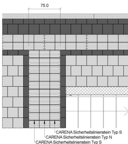
Bild 17: Anordnung von Aufmerksamkeitsfeldern mit einer Breite von 75 cm mit Steinen H = 6 cm
