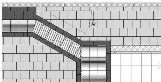
Bild 11: Anordnung bei ungenügender Breite für den sicheren Bereich
