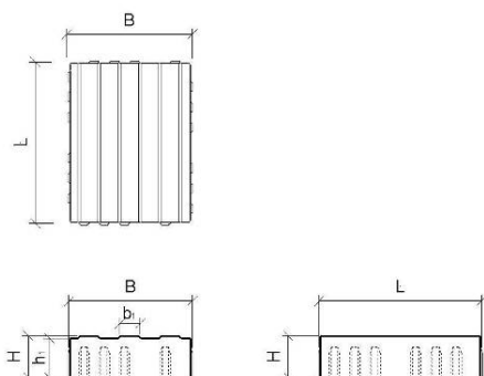
Bild 3: CARENA® Sicherheitslinienstein Typ N; H 6 cm
