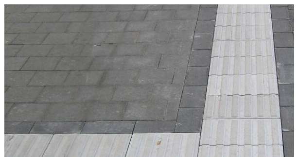
Bild 29: Ideale Anordnung von Passsteinen bei einem Anschluss an eine Sicherheitslinie
