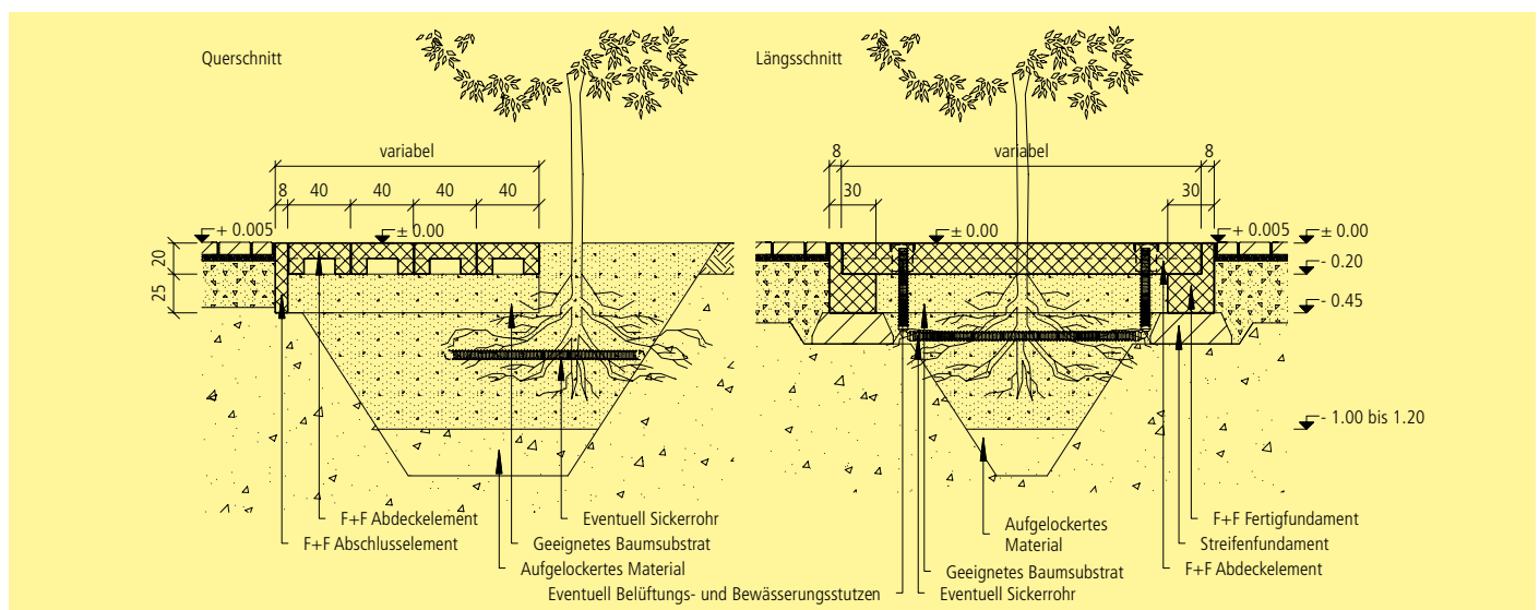
Einbauschema F+F Baumwurzelraumschutz als Wegbrücke mit Fertigteilfundament und einem Abschlusselement
