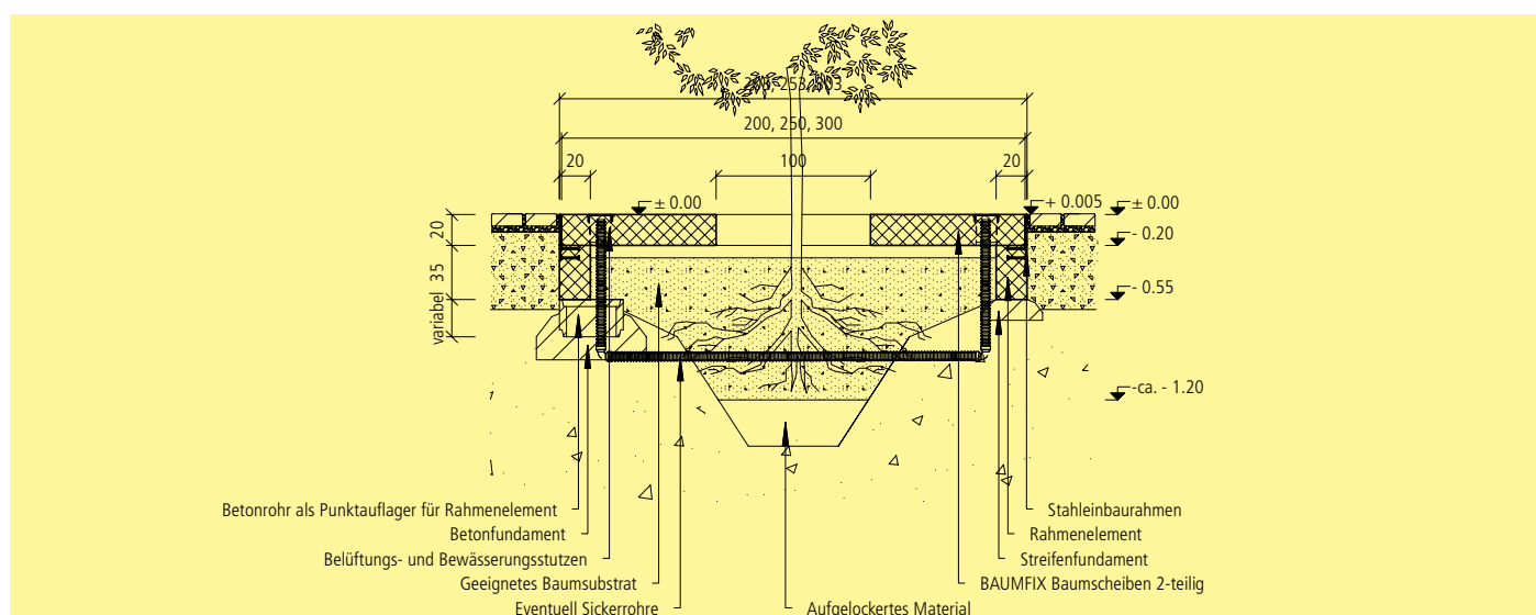
Einbauschema BAUMFIX® Baumscheiben mit Rahmenelement
