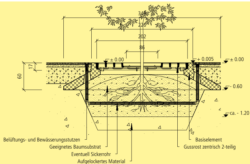
Einbauschema COPAL CUPOLA Baumwurzelraumschutz mit Gussrost
