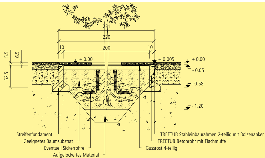
Einbauschema TREETUB Baumwurzelraumschutz mit Gussrost
