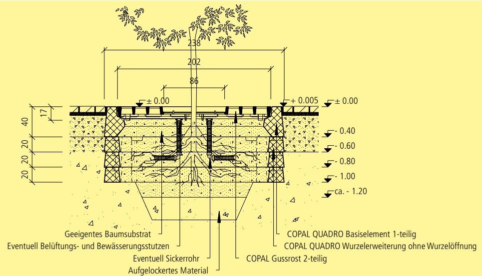
Einbauschema COPAL QUADRO Baumwurzelraumschutz mit Gussrost und Wurzelraumerweiterung ohne Wurzelöffnungen
