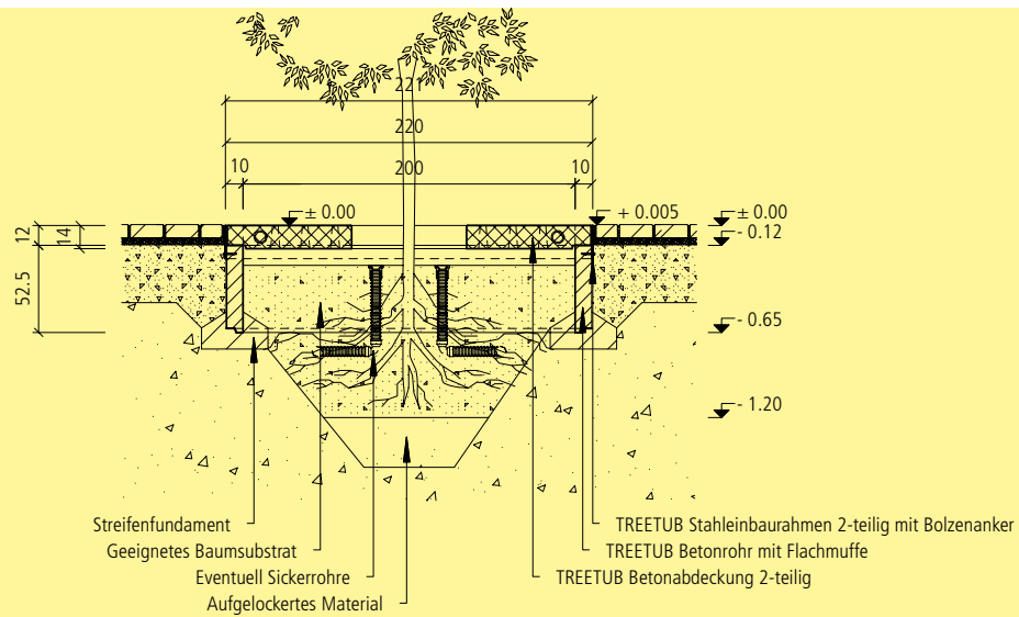
Einbauschema TREETUB Baumwurzelraumschutz mit Betonabdeckung
