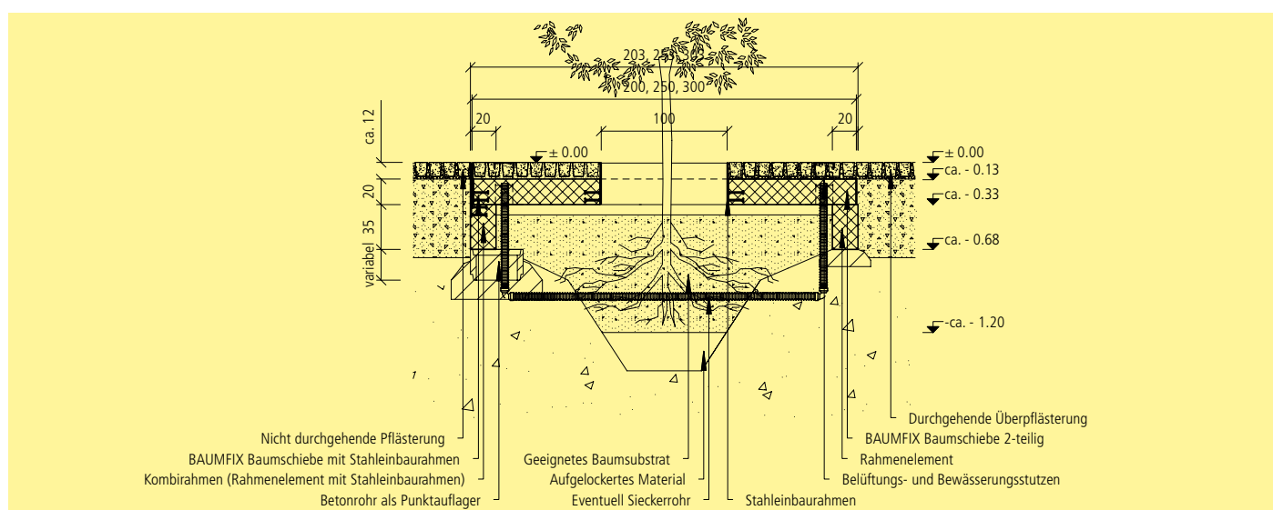
Einbauschema BAUMFIX® Baumscheiben mit Rahmenelement und Überpflasterung (Variante Unterflur)
