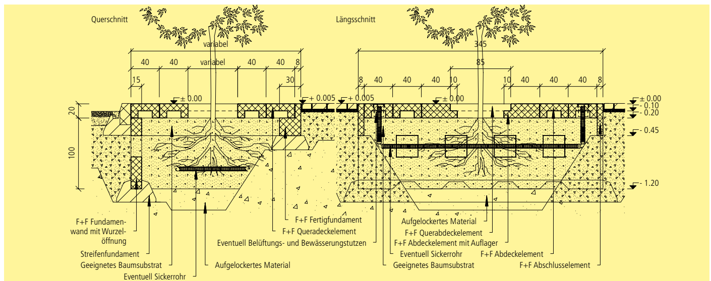
Einbauschema F+F Baumwurzelraumschutz mit Fundamentwand mit Wurzelöffnungen, Fertigteilfundament und Abschlusselement
