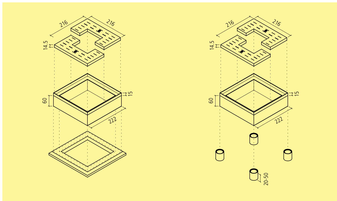
Kombination WILD Baumgruben
