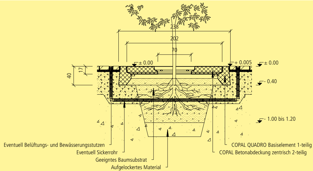
Einbauschema COPAL QUADRO Baumwurzelraumschutz mit Betonabdeckung zentrisch
