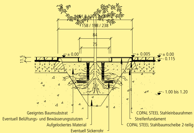
Einbauschema COPAL STEEL Stahlbaumscheibe mit Streifenfundament
