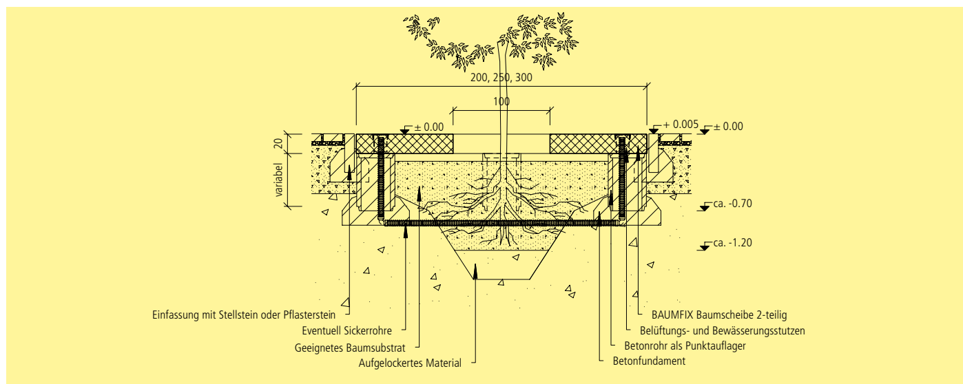
Einbauschema BAUMFIX® Baumscheiben auf Punktaufleger (z.B. Betonrohre DN 300)
