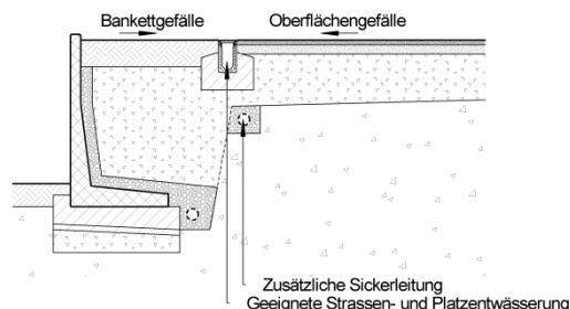
Bild 29: Zusätzliche Entwässerung
