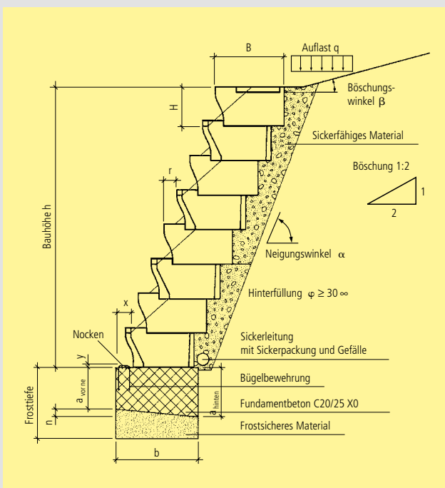
Böschungselemente Aufbau
