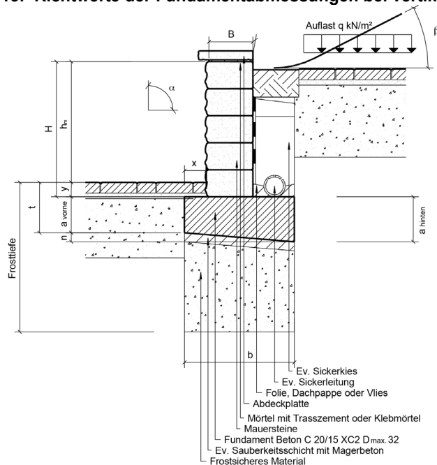
Bild46: Vertikaler Maueraufbau
