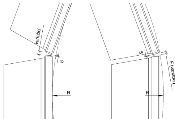
Bild 14: Klaffende Fugen bei Kurven
