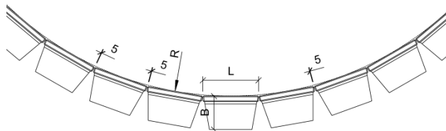
Bild 14: Klaffende Fugen bei Kurven
