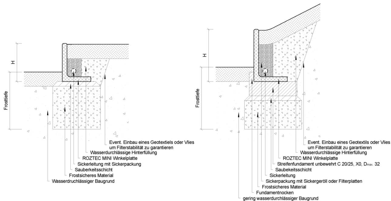
Bild 12: Schematische Darstellung des Aufbaus mit oder ohne Streifenfundament
