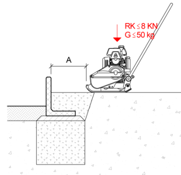
Bild 10: Lastfall F
