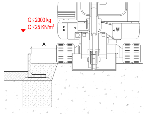
Bild 11: Lastfall G
