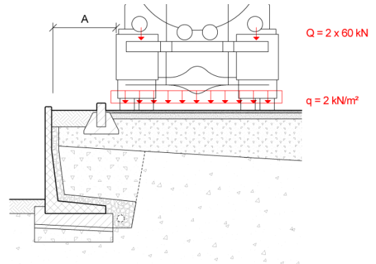
Bild 14: Lastfall C4
