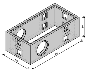
Type 2.1, B 120cm L 240cm H 80cm
