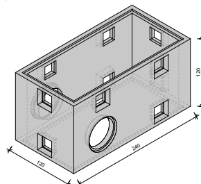
Type 2.1, B 120cm L 240cm H 120cm
