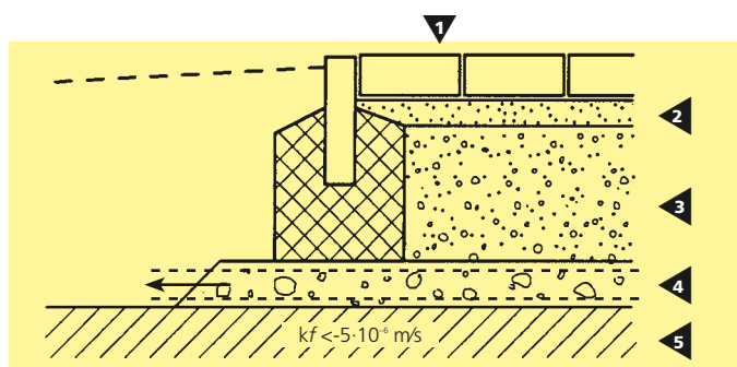
Wasserablenkung oberhalb des Planums bei nicht ausreichend versickerungsfähigem Untergrund Darstellung 22
