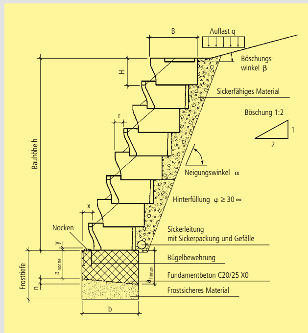
Böschungselemente Aufbau
