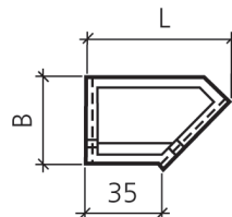
Bild 10: ECKELEM. Innenecke links (einspringend)
