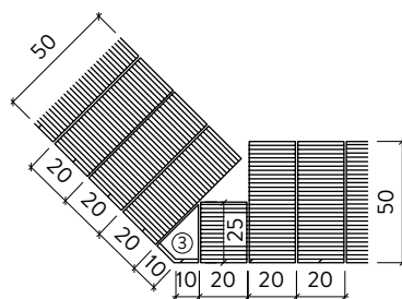
Lagen 2, 4, 6 usw.
