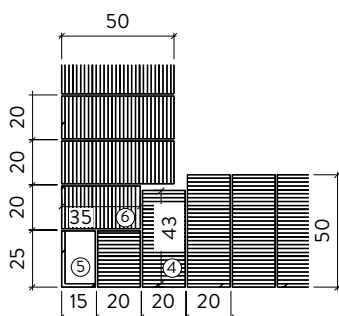
Lagen 1, 3, 5 usw.
