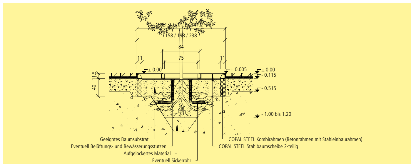
Einbauschema COPAL STEEL Stahlbaumscheibe mit Kombirahmen
