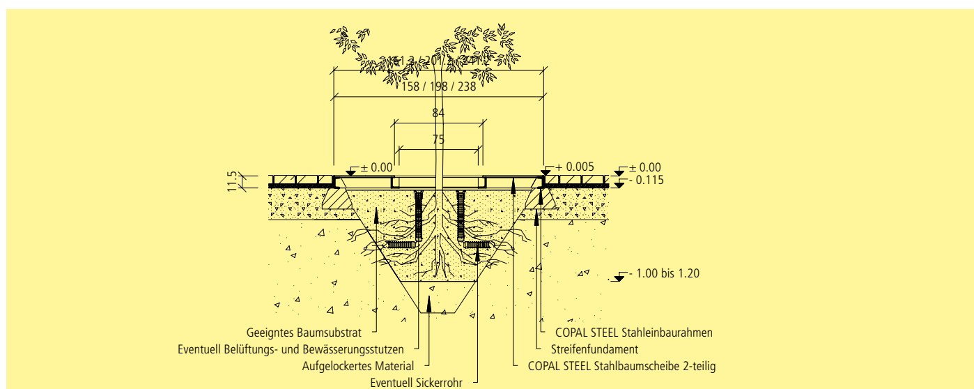
Einbauschema COPAL STEEL Stahlbaumscheibe mit Streifenfundament
