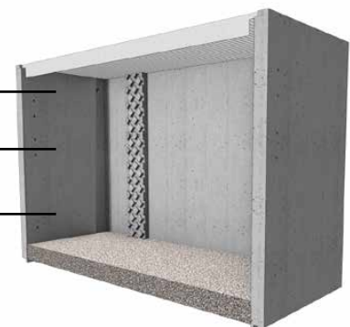
Schematischer Schnitt AMFIX® Amphibienausstieg eingebaut in einem Lichtschacht
