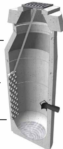
Schematischer Schnitt AMFIX® Amphibienausstieg eingebaut in einem Strassenablauf
