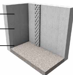
Schematischer Schnitt AMFIX® Amphibienausstieg eingebaut in einem Regenbecken
