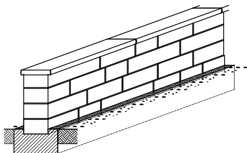
Bild 25: Freistehende Mauer
