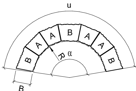
Bild 31: Optimale Muffenbildung
