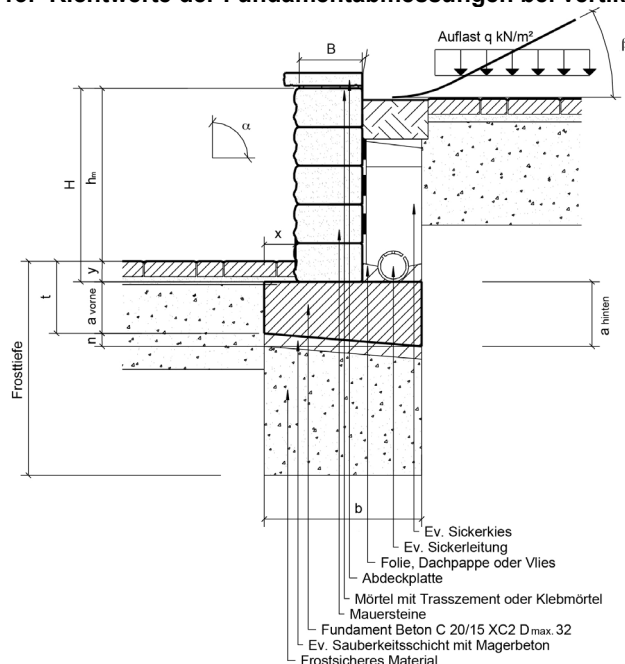
Bild46: Vertikaler Maueraufbau
