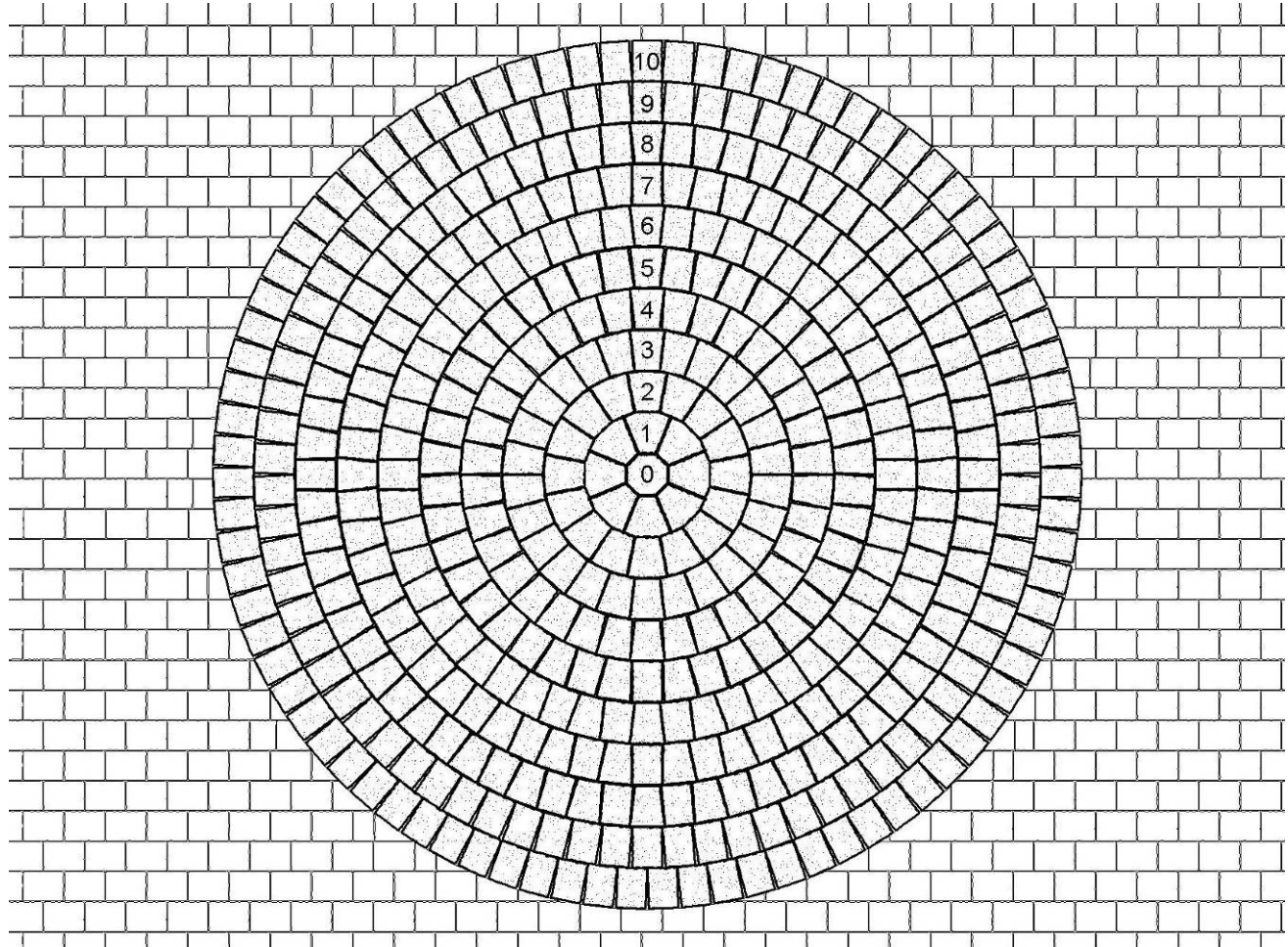
Verlegebild 19: Kreisverband mit TEGULA® Pflaster- und Kreissteinen
