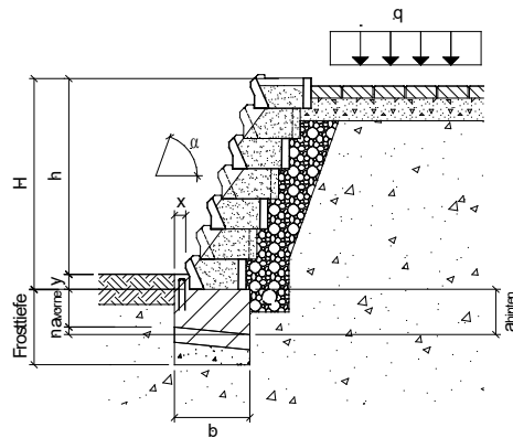
Max. Bauhöhe Elementhöhe Kronenrücksprung Fundamenthöhe Nockenhöhe y = Einbindtiefe Element Nockenabstand Einbindtiefe (Fundament) vorne / hinten Sohlenneigung Fundamenthöhe Fundamentbreite Anzahl Lagen Steine h cm H cm r cm a vorne cm y cm x cm t cm n cm a hinten cm b cm Stk. 90 100 28 20 5 10 25/30 5 25 55 5 110 120 35 25 5 10 30/35 5 30 60 6 150 160 52 25 5 15 30/40 10 35 75 8
